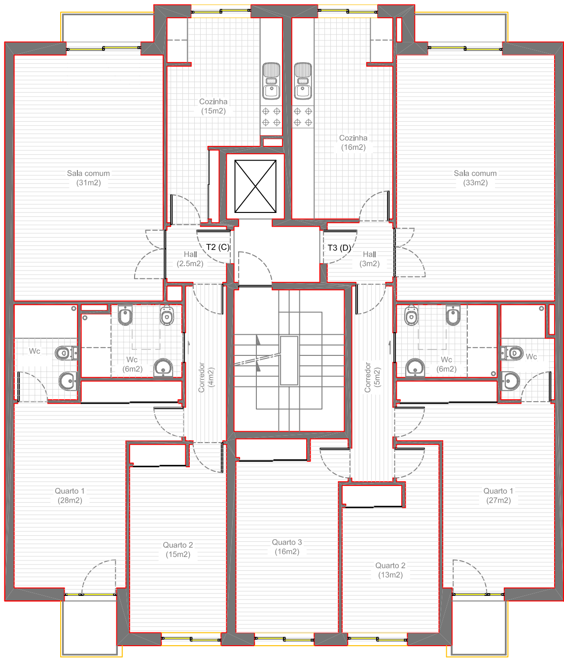
Lote de 15m. Escala=1:100. 1º andar
